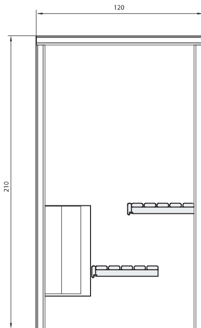
Sezione laterale
